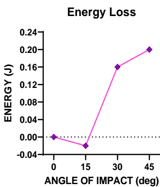
Рис. 4. Потеря энергии (Energy Loss — потеря энергии; Energy, J, — энергия, Дж; Angle of Impact, deg, — угол встречи, град.).
