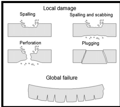
Рис. 1. Локальные повреждения и глобальное разрушение [4] (Local damage — локальное повреждение; Spalling — скалывание; Spalling and scabbing — скалывание и выкрашивание; Perforation — перфорация; Plugging — разламывание; Global failure — глобальное разрушение).
