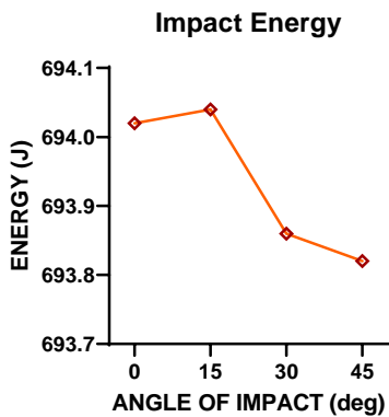
Рис. 3. Энергия удара (Impact Energy — энергия удара; Energy, J, — энергия, Дж; Angle of Impact, deg, — угол встречи, град.).
