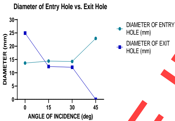
Рис. 7. Диаметр входного отверстия в сравнении с выходным отверстием (Diameter of Entry Hole vs. Exit Hole — диаметр входного отверстия в сравнении с выходным отверстием; Diameter, mm, — диаметр, мм; Angle of Incidence, deg, — угол падения, град.; Diameter of Entry Hole, mm, — диаметр входного отверстия, мм; Diameter of Exit Hole, mm, — диаметр выходного отверстия, мм).
