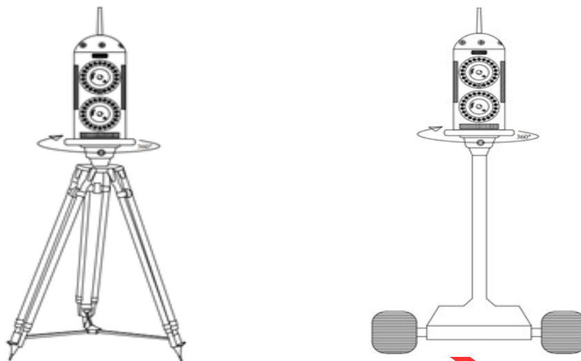
Рис. 1. Модульный комплект (со штативом и в передвижном виде).
