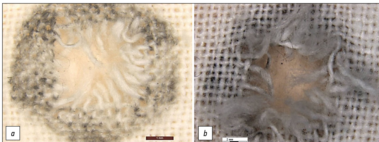
Рис. 4. Повреждение сухой бязевой мишени, причинённое выстрелом из пистолета Glock 17 с расстояния 40 см: a — лицевая сторона мишени; b — изнаночная сторона мишени.
