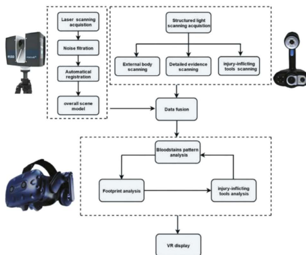
Рис. 3. Схема интегрированной платформы 3D-сканирования [18]. Fig. 3. Scheme of the integrated 3D scanning platform [18].
