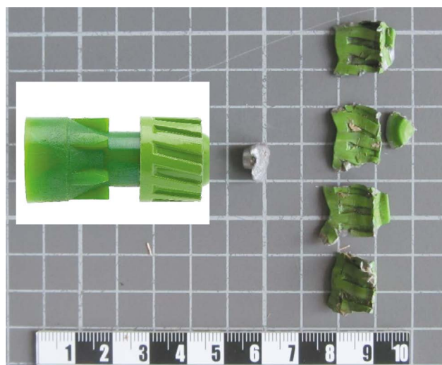
Рис. 1. Пуля к патрону «УНО 35Э» до (слева) и после (справа) взаимодействия с мишенью.
